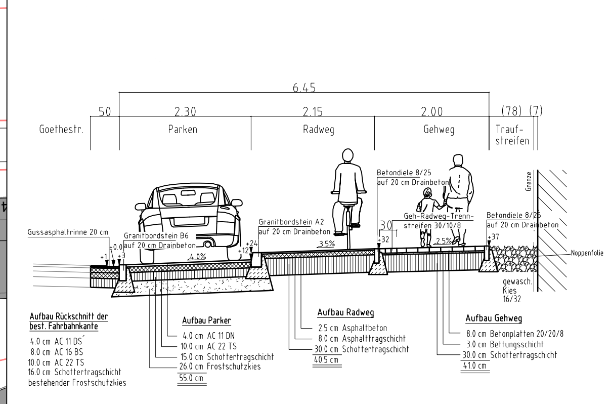
Regelquerschnitt Goethestraße mit Parker
