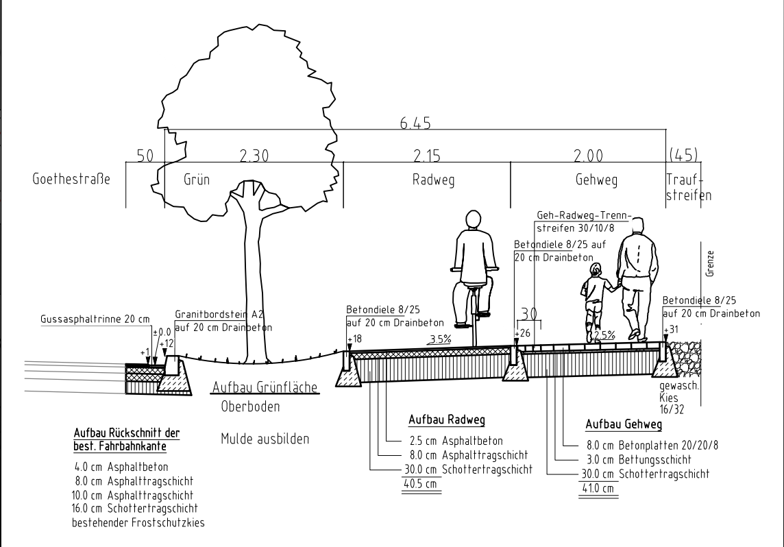
Regelquerschnitt Goethestraße mit Grünfläche
