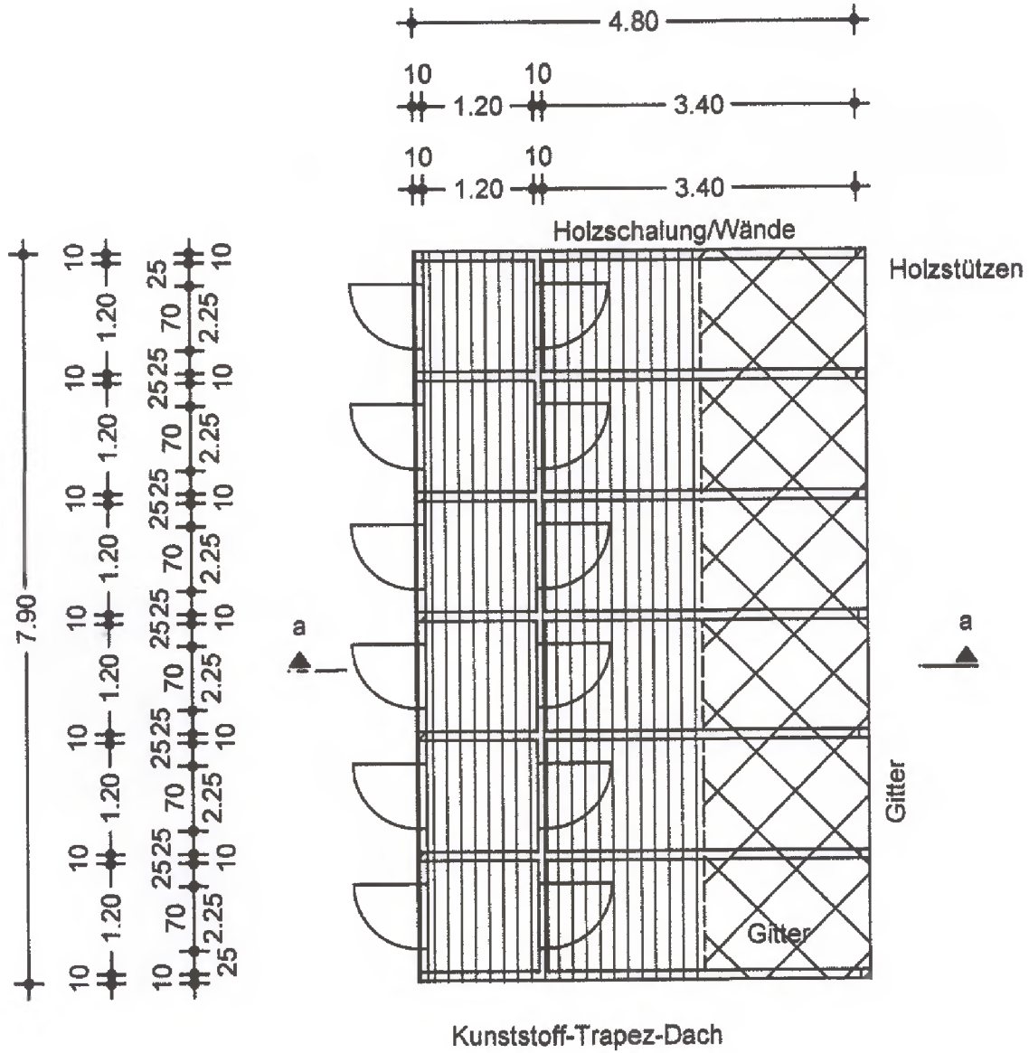
Voliere Grundriss
