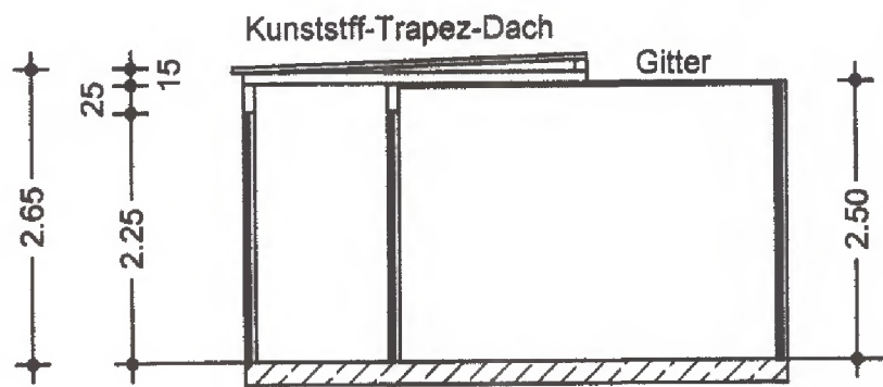
Voliere Schnitt
