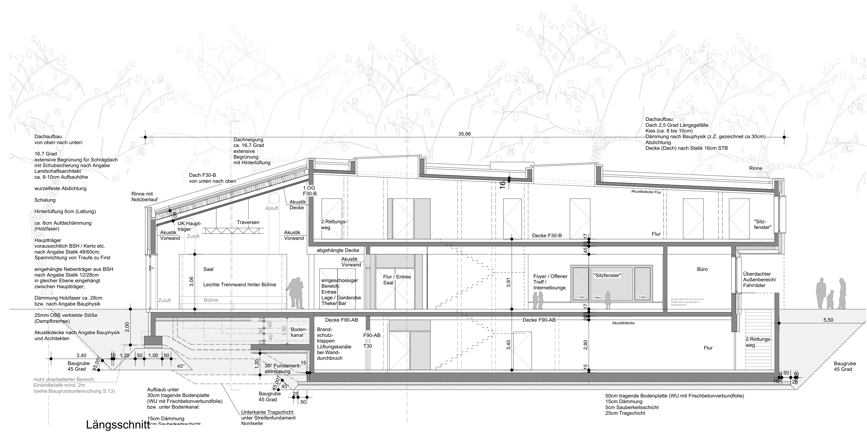
Längsschnitt
