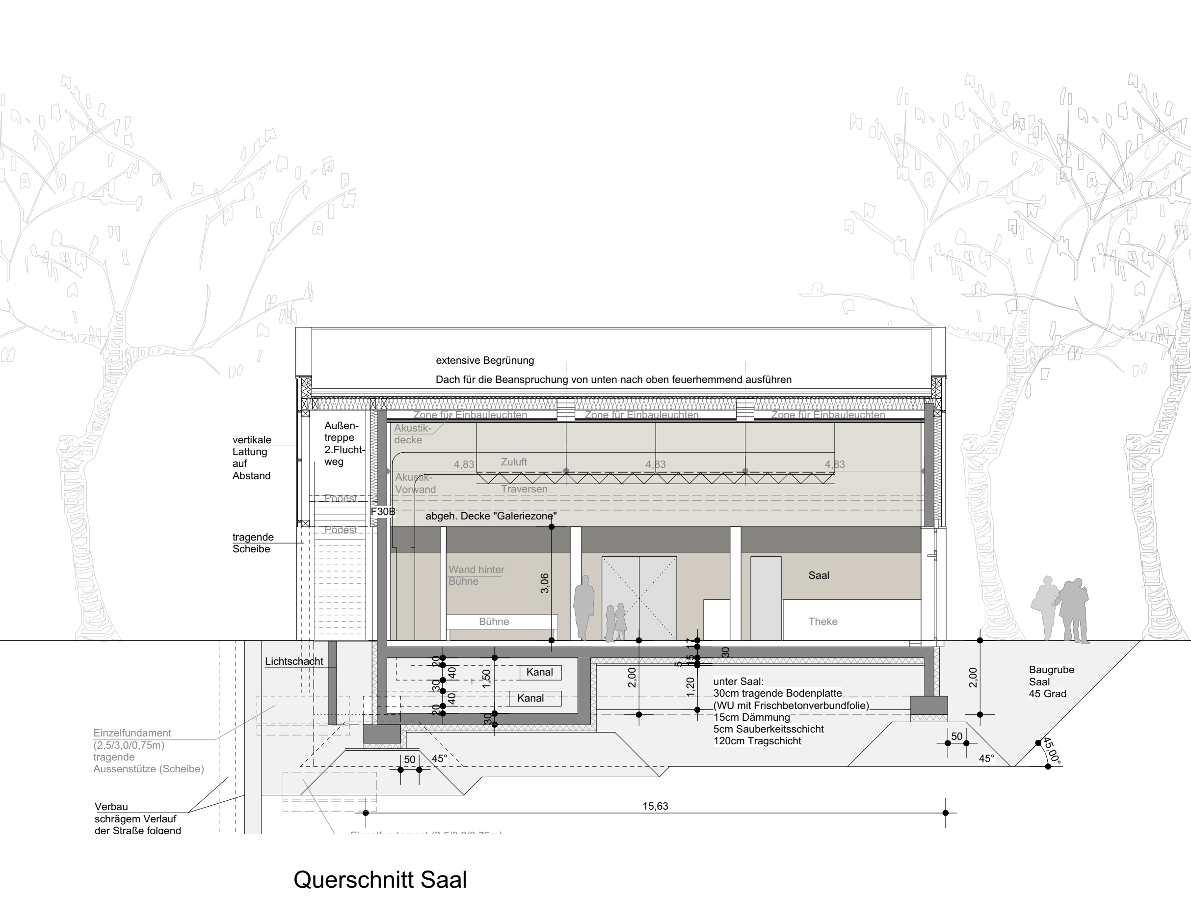
Querschnitt Saal
