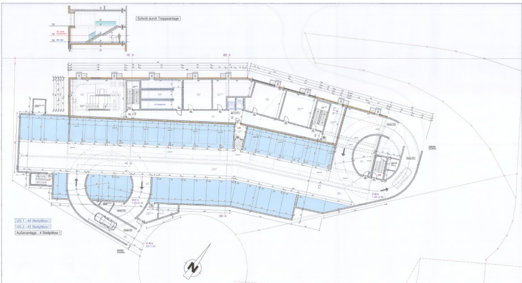
Grundrisse UG 1
