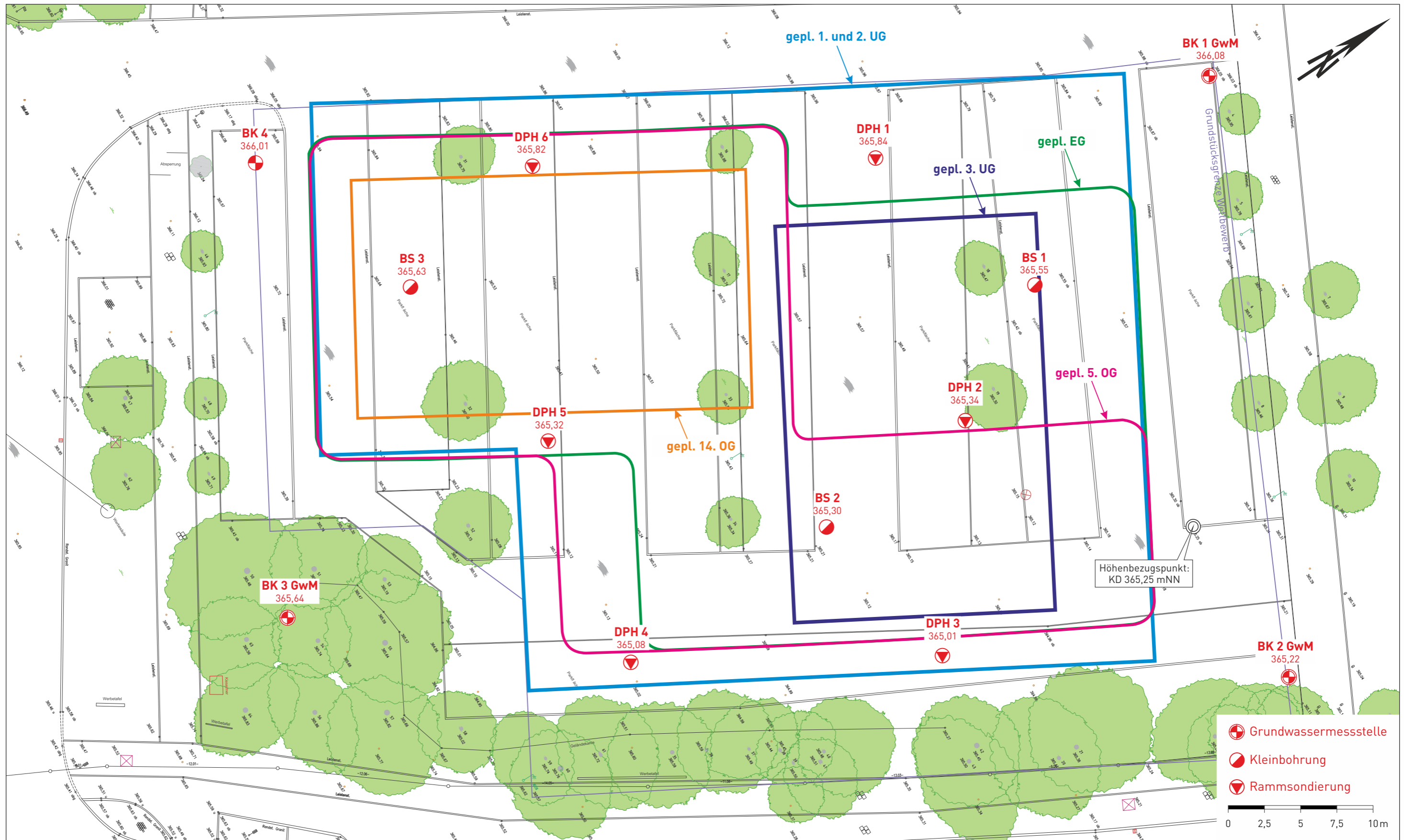
Lageplan mit Lage der Erkundungspunkte
