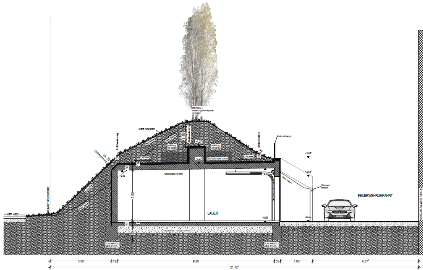
SCHNITT 1-1 M 1:50
