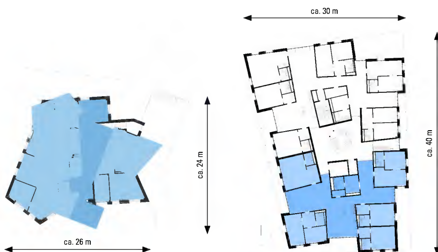
Abb. 102: Tiefe der Baukörper: Grundrisse der Cluster-Wohnungen von wagnisART , München (links) und mehr als wohnen , Zürich (rechts)
