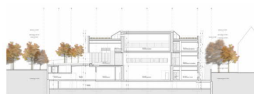
Schnitt DD
