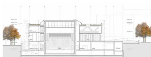
Schnitt CC
