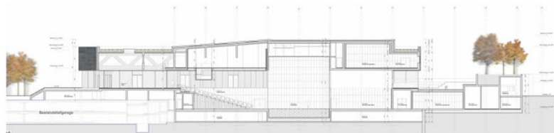
Schnitt AA
