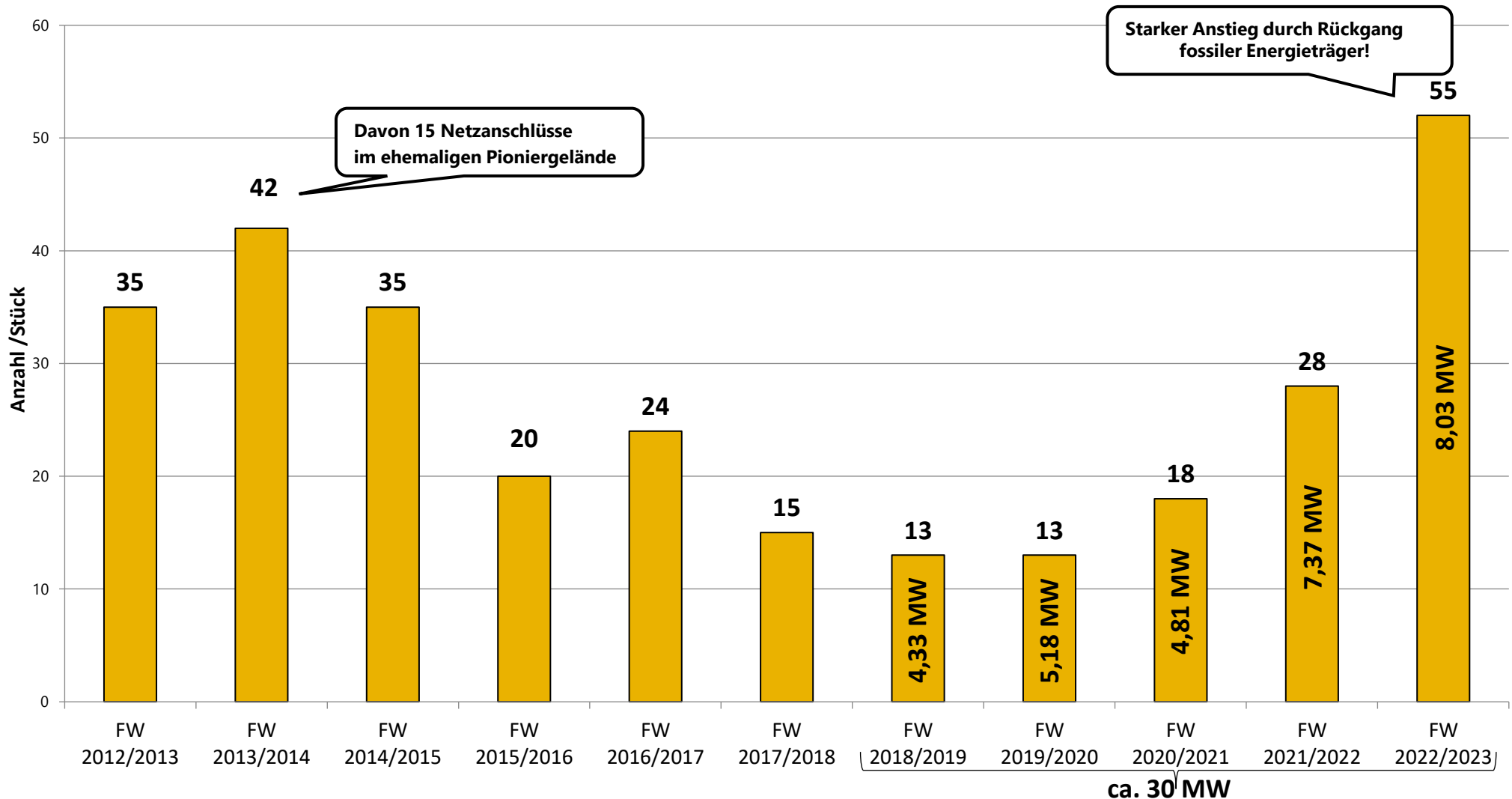
Anzahl Fernwärmenetzanschlüsse WJ 2013-2023 (Stand 30.09.2023)
