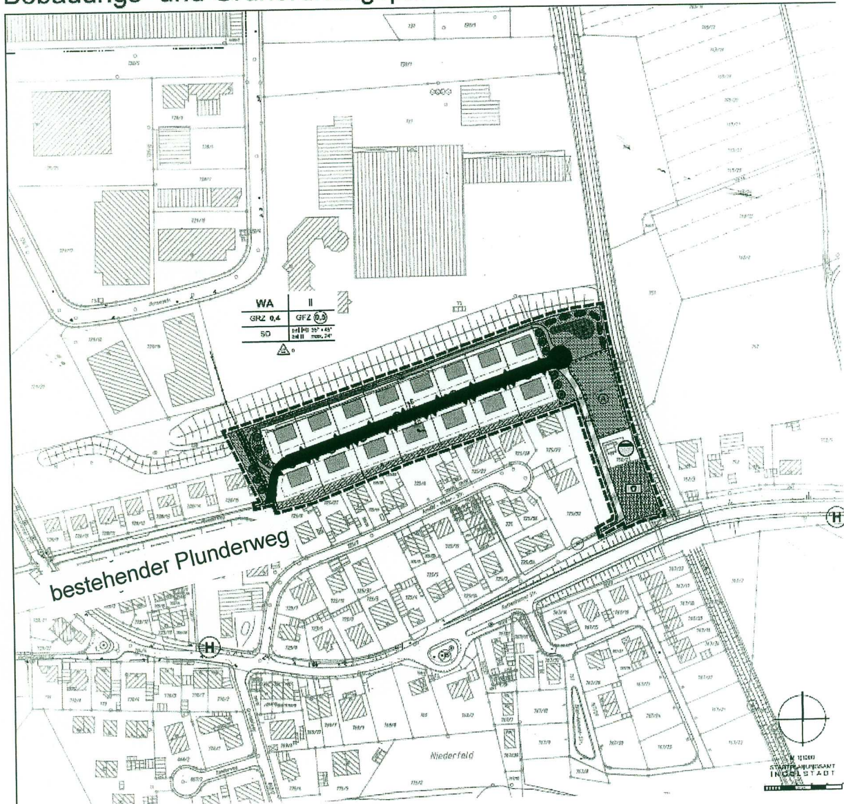
Bebauungs- und Grünordnungsplan Nr. 145 H - "Niederfeld"
