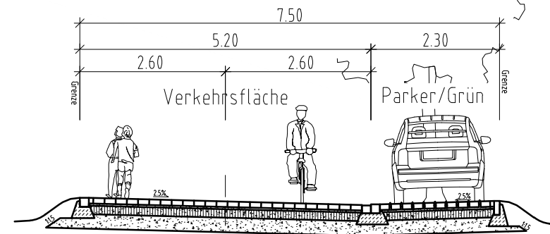
Schnitt A-A Verkehrsberuhigte Bereiche
