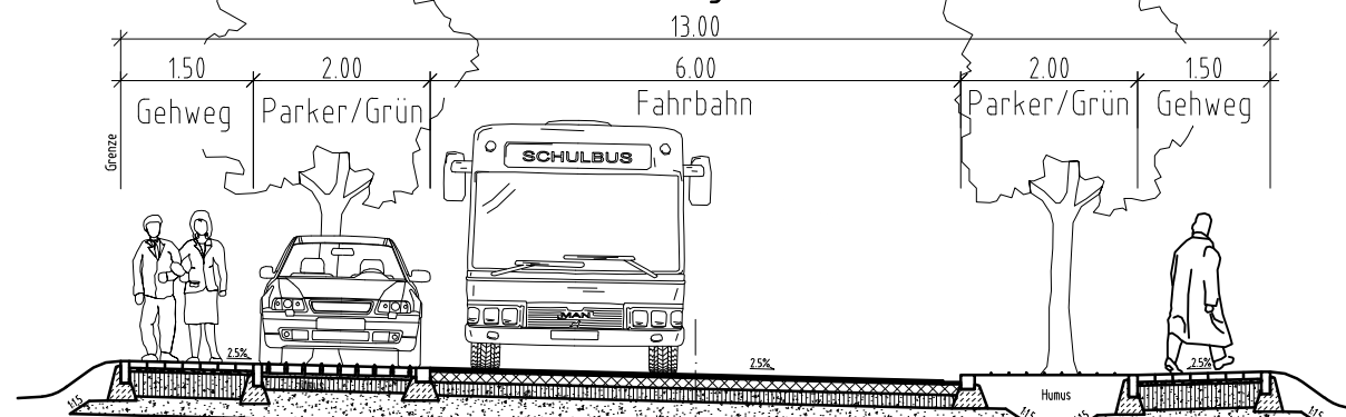
Schnitt B-B Jurastraße/Steigerwaldstraße
