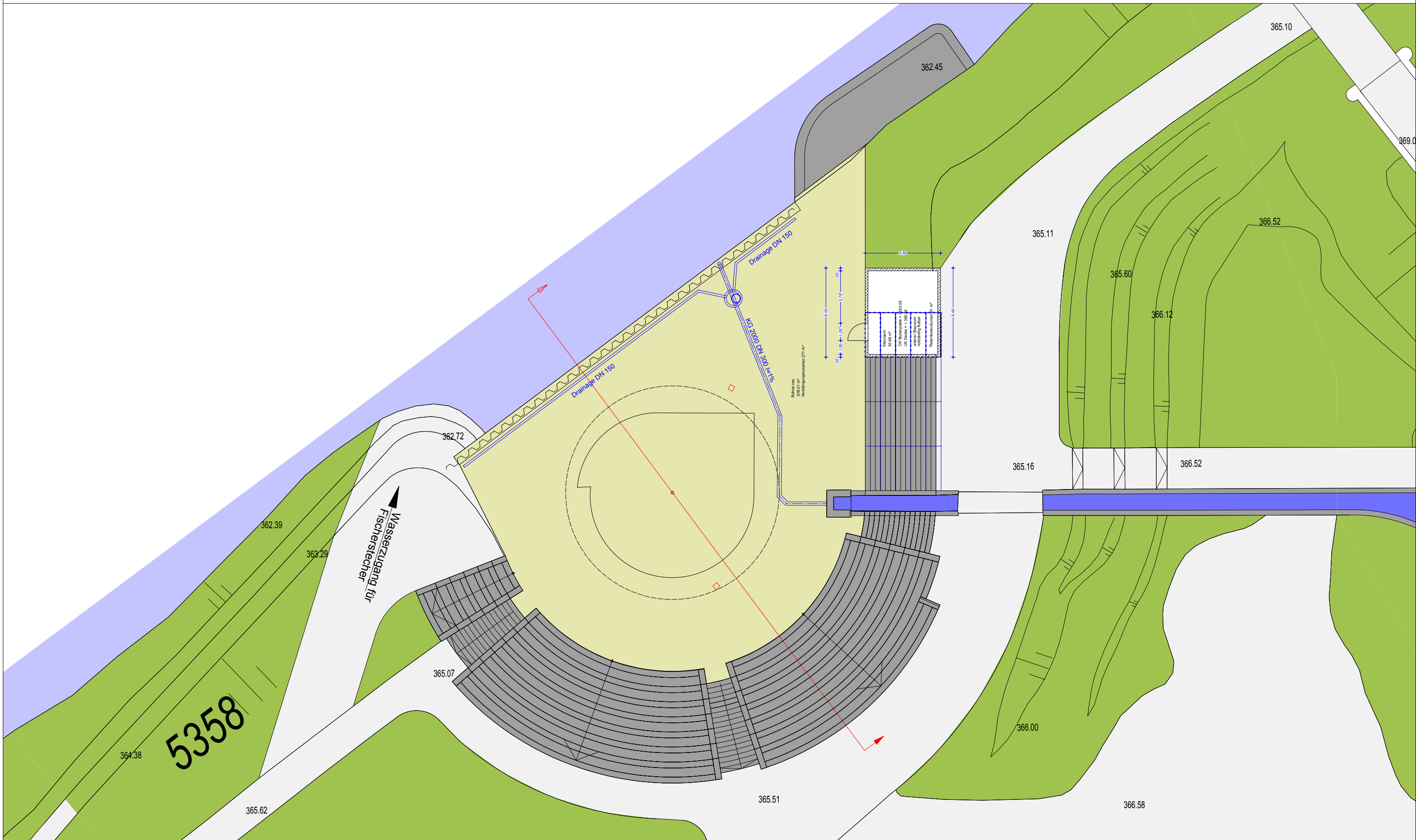
Vorentwurf Erweiterung der Donaubühne Grundriss M. 1 : 250
