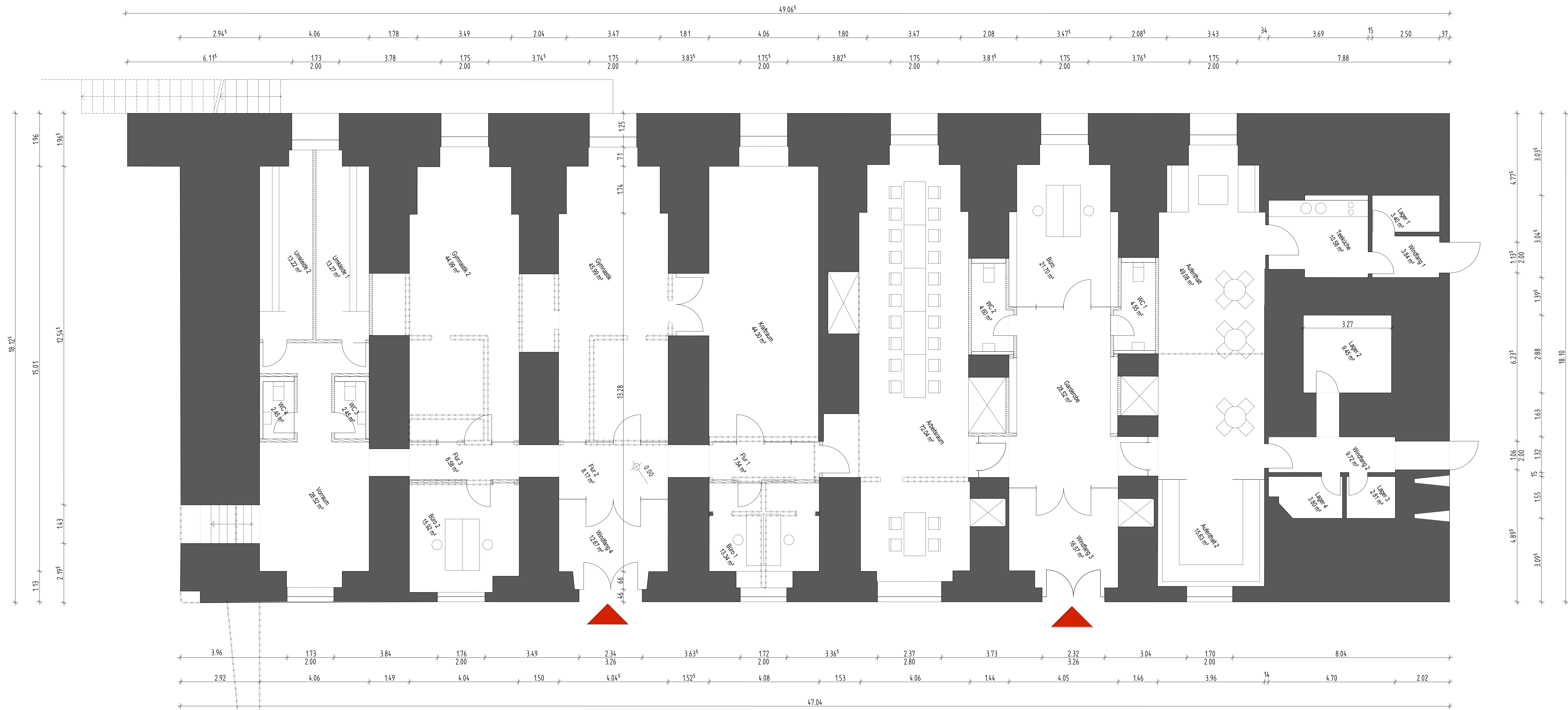
GRUNDRISS BATTERIE M.:1:50
