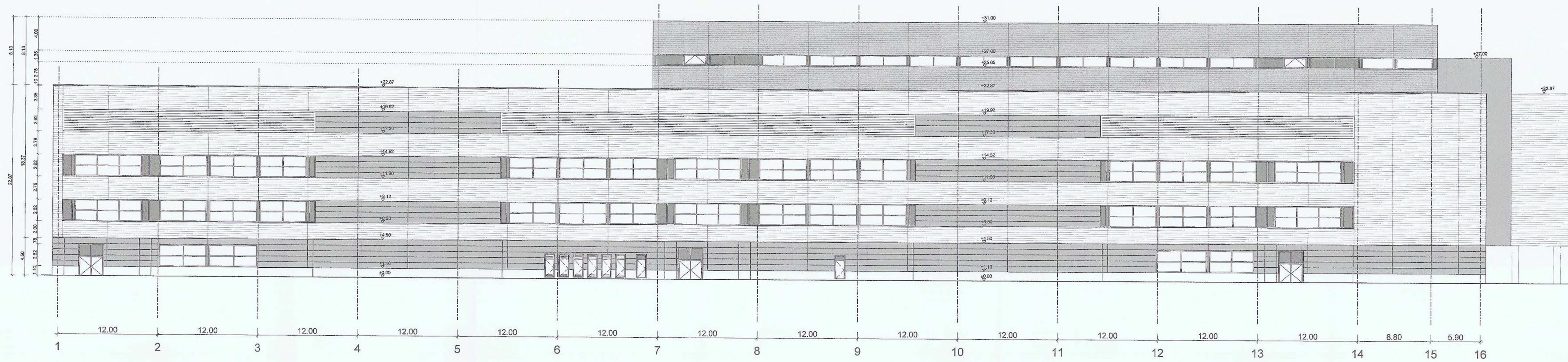
Ansicht Süd-West
