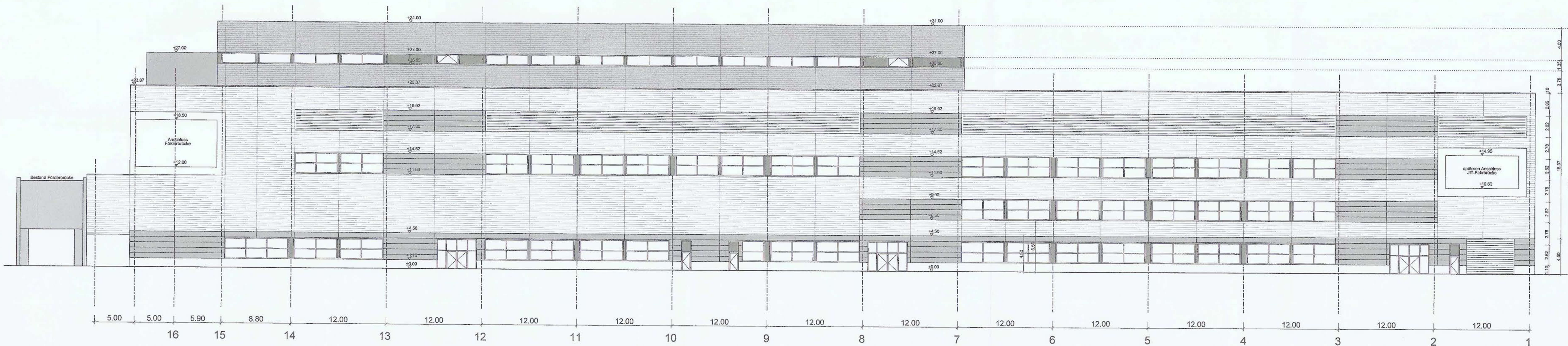
Ansicht Nord-Ost
